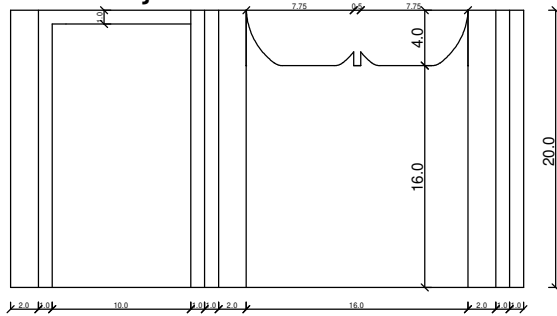
Przekrój A-A
